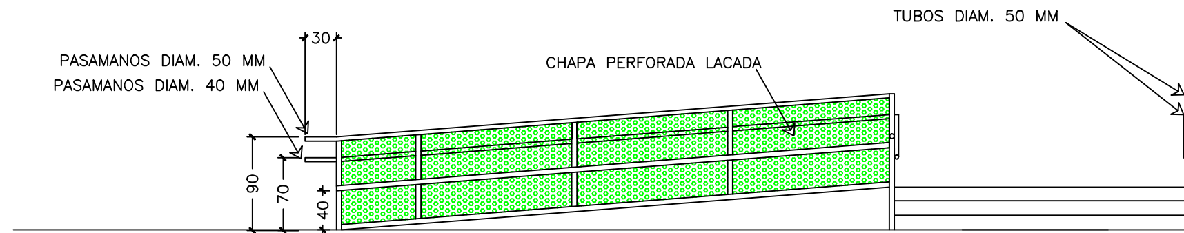
ALZADO
